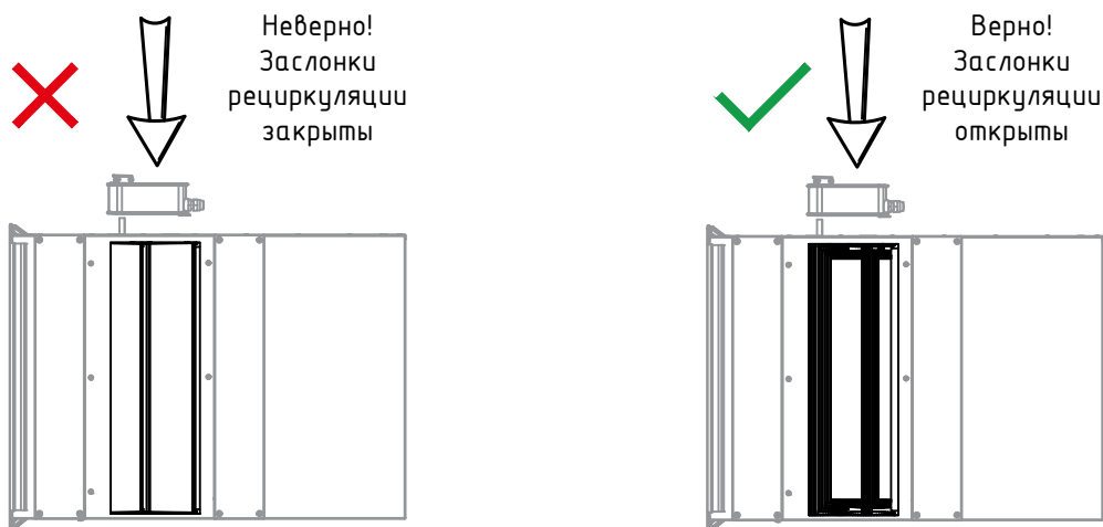
Рис. 3. Положение дроссельных заслонок перед монтажом сервопривода
