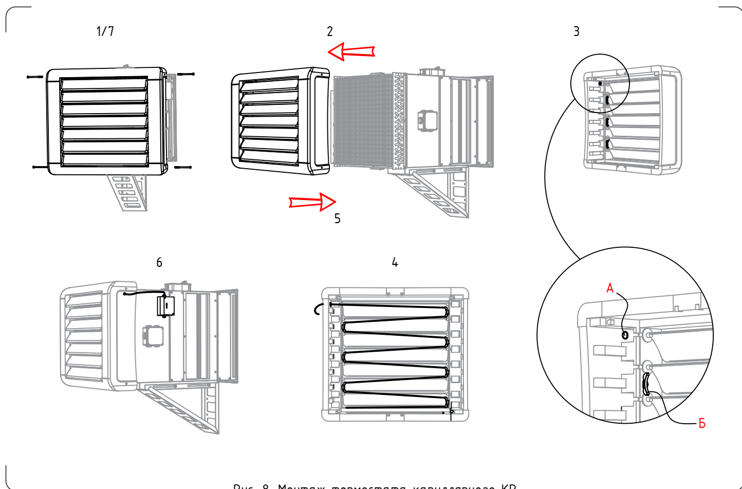
Рис. 8. Монтаж термостата капиллярного КР
