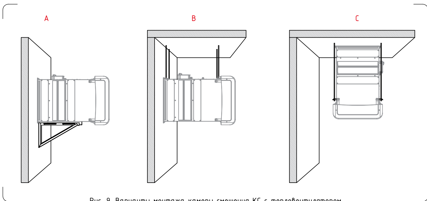
Рис. 9. Варианты монтажа камеры смешения КС с тепловентилятором
