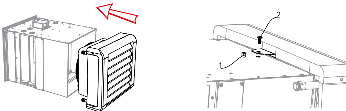
Рис. 6. Крепление тепловентилятора к камере смешения КС
