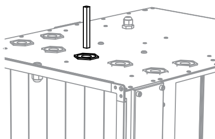
1. Установка оси сервопривода
