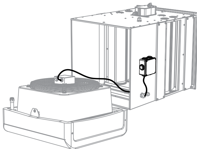
Рис. 5. Протяжка провода через кабельный ввод
