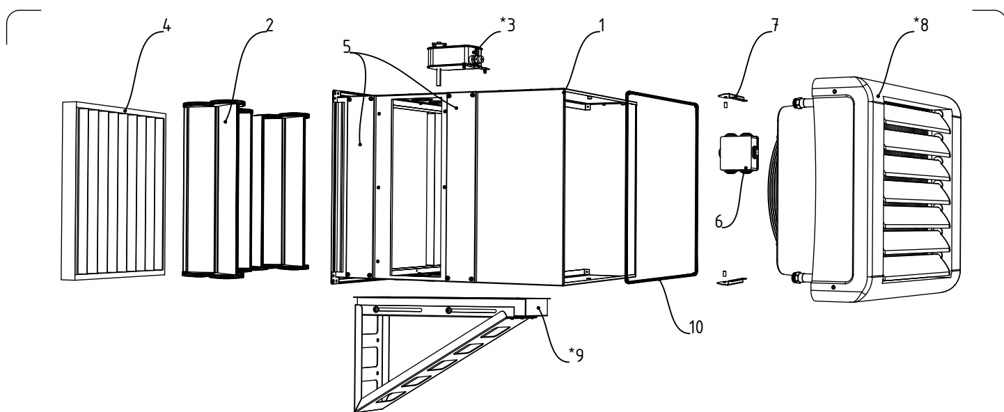
Рис. 2. Составные элементы камеры смешения ГРЕЕРС КС и тепловентилятора
