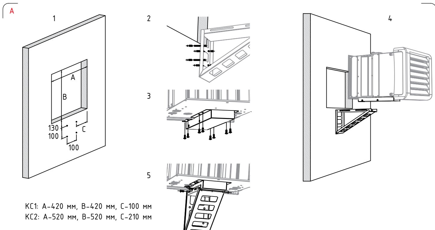
Рис. 10. Установка камеры смешения с тепловентилятором на монтажную консоль
