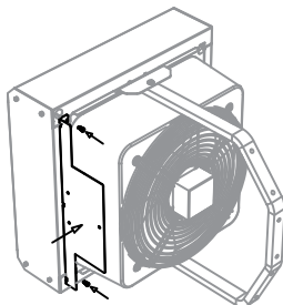
Рис. 7. Перенос крепления блока БПУ-ЕС у ГРЕЕРС ЕС
