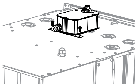
2. Установка сервопривода
