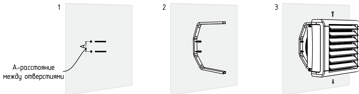
Рис. 5. Монтаж консоли
