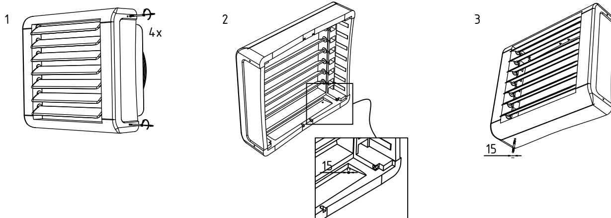
Рис. 2. Установка штуцера на передней части корпуса
