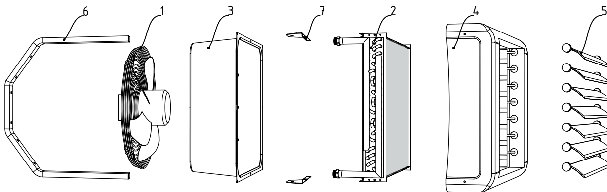
Рис. 1. Составные элементы тепловентилятора ГРЕЕРС ВС
