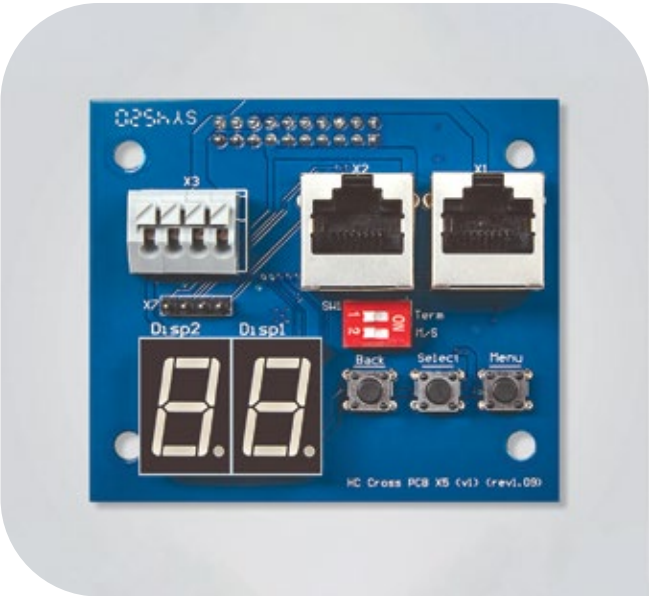
Низковольтное управление, подключение кабелем RJ-45
