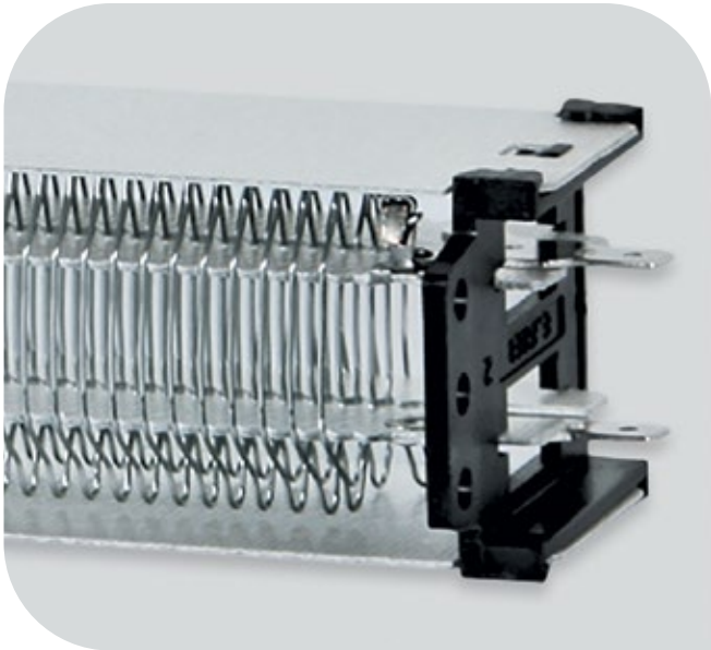
Нагревательный элемент на основе термостойкого каркаса
